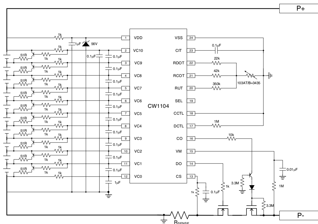
10 串带均衡功能应用电路
