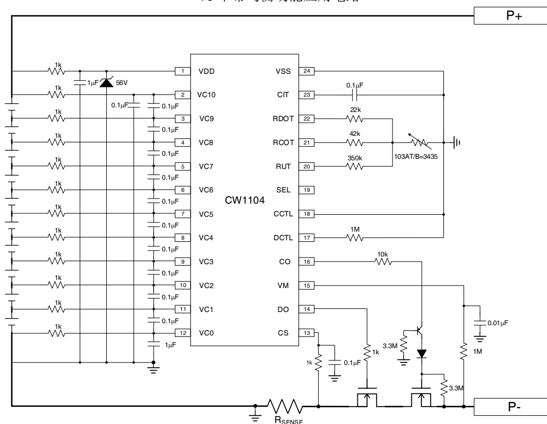
10 串不带均衡功能应用电路
