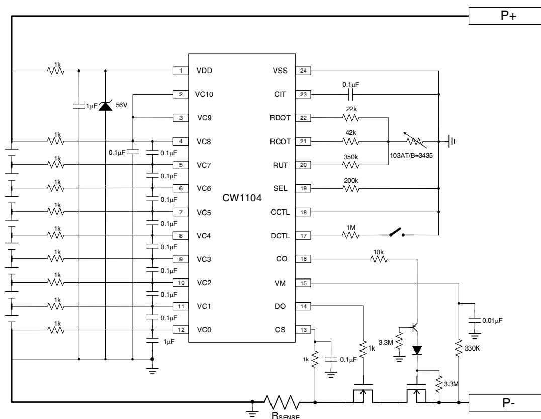
8 串同口应用电路（电子锁）
