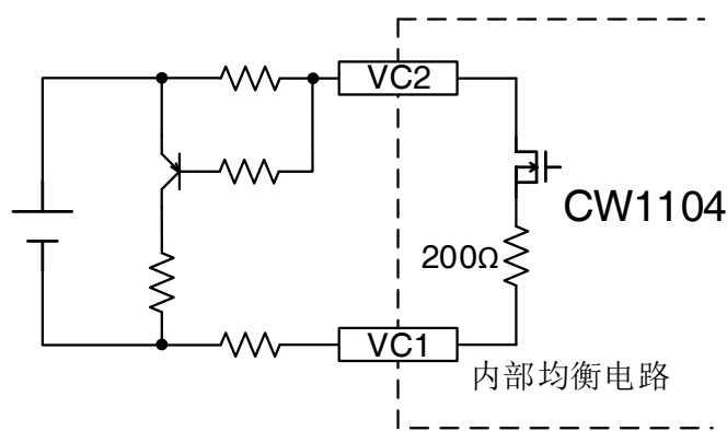
均衡功能示意图
