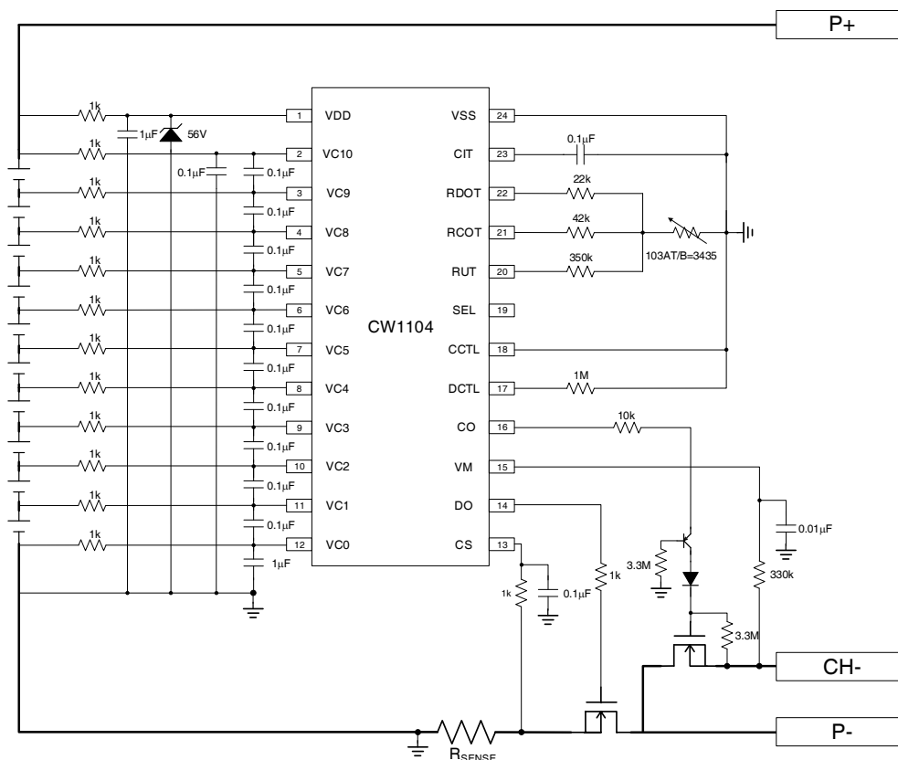
10 串异口应用电路 (CH-)
