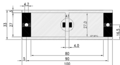
(圖三 Fig3)For 30A~40A
