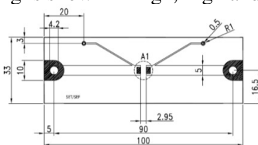
(圖二 Fig2)For 20A~25A
